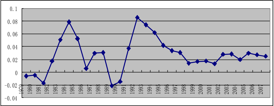
图 2: 各年度 TFP 增长率
