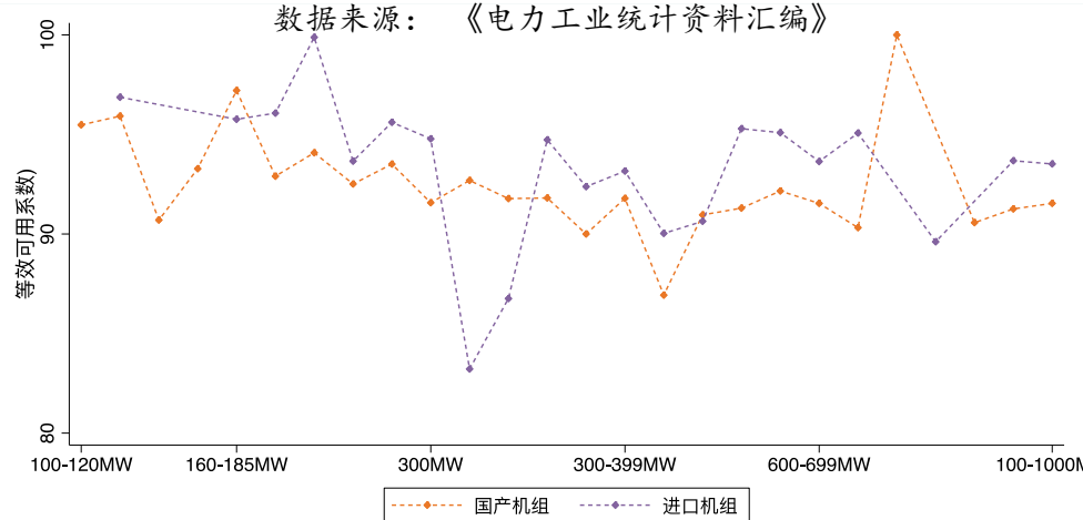
图 2021年全国火电100兆瓦及以上容量机组等效可用系数
