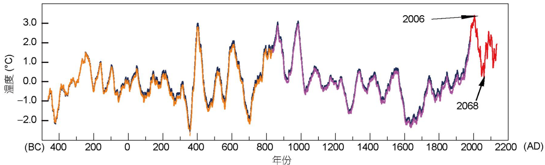
图3 温度变化的千年尺度周期 资料来源：刘禹等（2011）
