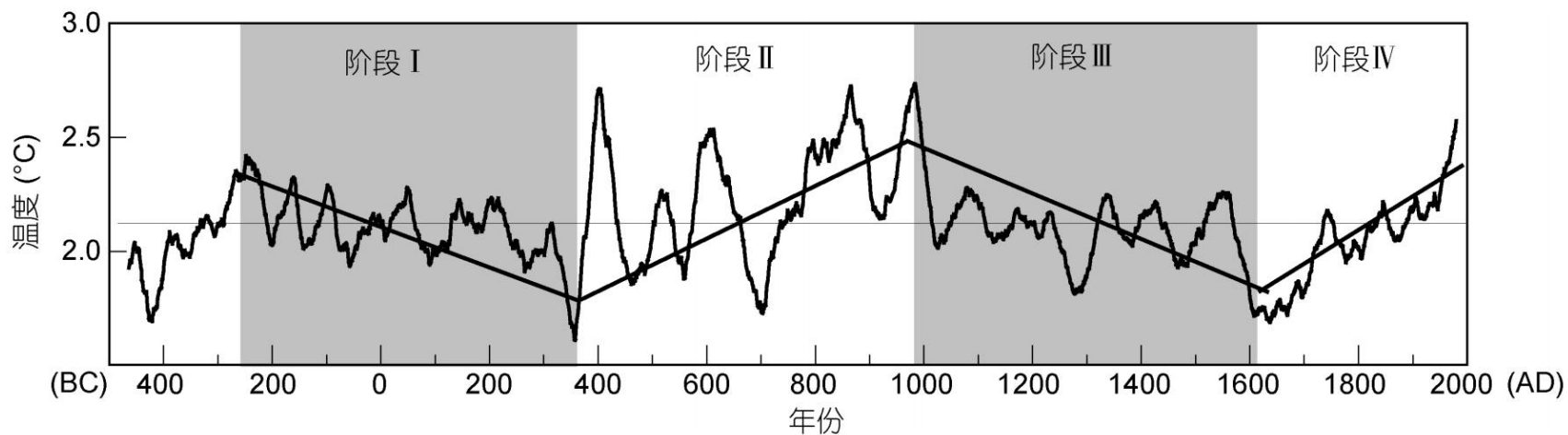
图3 温度变化的千年尺度周期 资料来源：刘禹等（2011）
